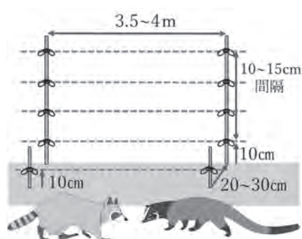
4段張り及びトリップ方式
