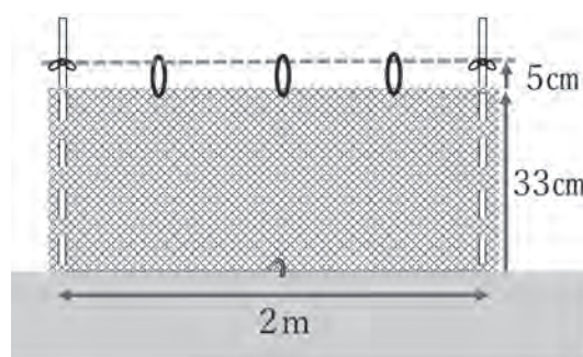
楽落くん設置方法（イノシシ対策としても活用されている方法）
